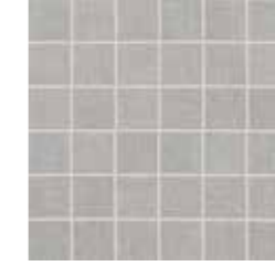
MIKTOZCE MIKASA MOS. QUAD SU RETE CENERE 205 MQ 30x30 12"x12" Spessore thickness 9,5 mm PCS/BOX 9,00 MQ/BOX 0,81 KG/BOX 14,70 MQ/pallet 29,16 BOX/pallet 36
